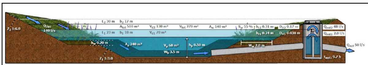
Föreslagen utformning på dagvattendamm (Kodeda, 2023-12-04)
