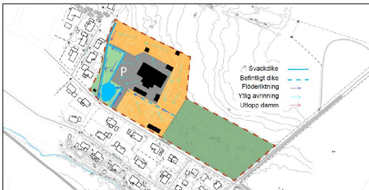
Föreslagen dagvattenlösning (Kodeda, 2023-12-04).
